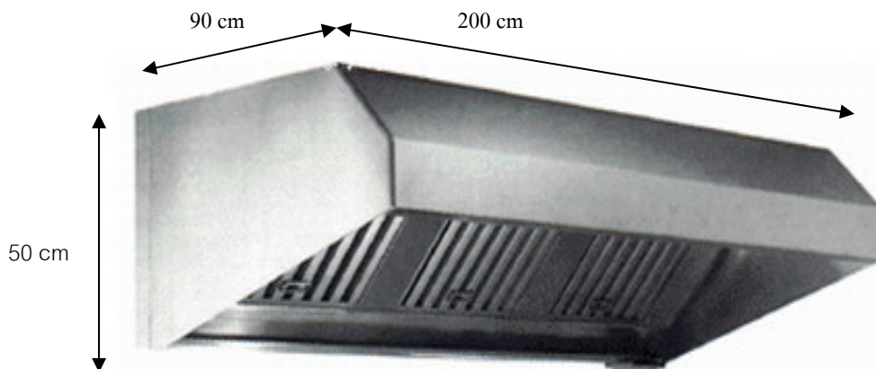
รูปแบบของ EXHAUST HOOD
